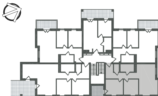
USYTUOWANIE LOKALU W BUDYNKU
