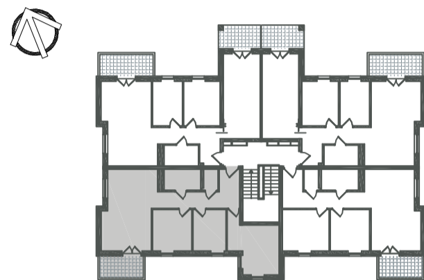
USYTUOWANIE LOKALU W BUDYNKU
